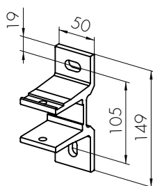
Väggfäste
