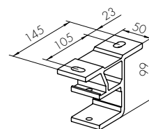
Takfäste
