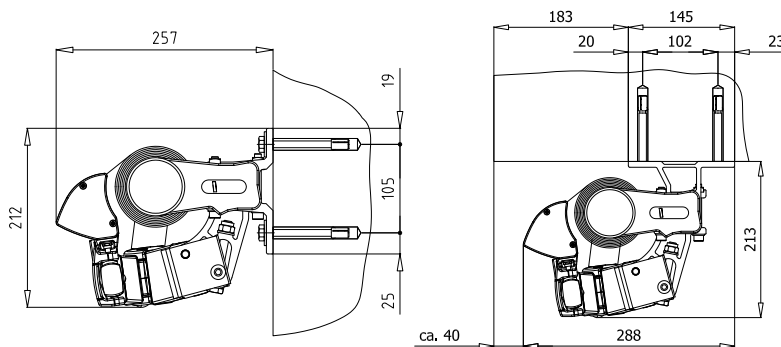
Väggmontage
