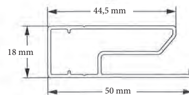
Vägghmontering
