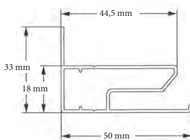
Nischmontering
