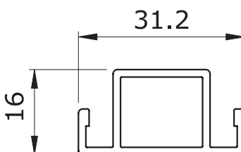
Mellanregel
