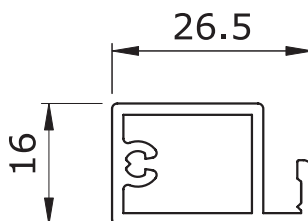
Dörrprofil
